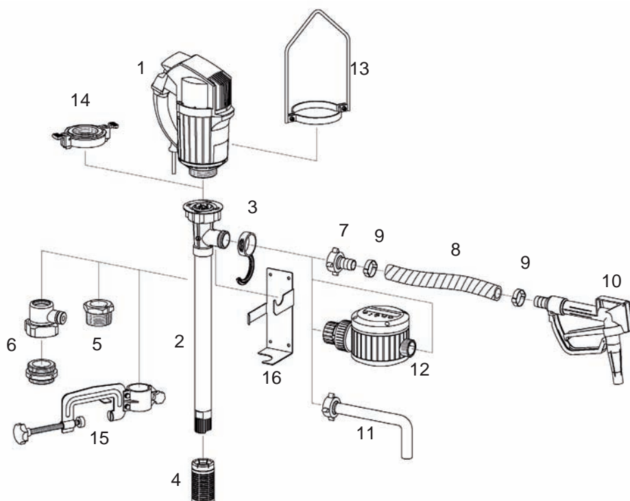
Fig. 1: Conception de la pompe non-antidéflagrante (avec composants)
